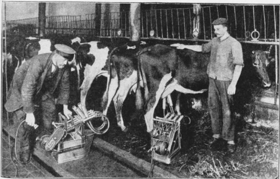
Melken mit Maschinen. Seit einem Menschenalter beschäftigt sich die Technik mit dem Gedanken des mechanischen Melkens, das bisher eine unbestrittene Arbeit der Hand war. Die hier abgebildeten Melkmaschinen verdreifachen die Leistung des Handmelkens. (Atlantil)
