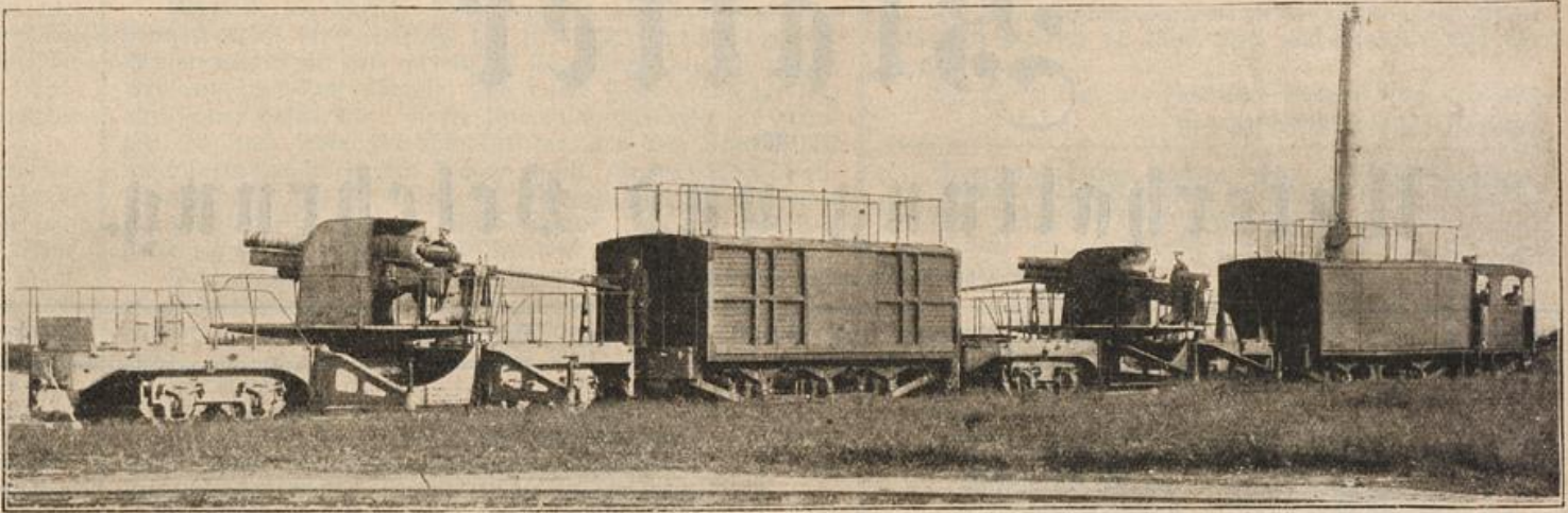
Eine neue fahrbare Batterie für die Küstenverteidigung. (S. 64)
