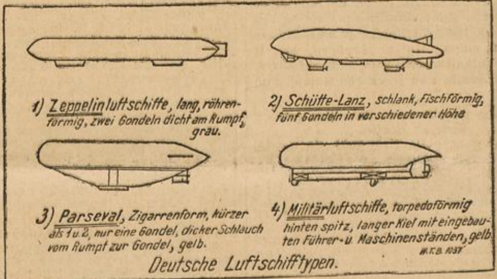
Deutsche Luftschiffotypen.
