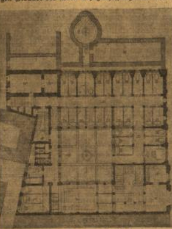
Erdgeschoß-Grundriß des 1867 erbauten Schützenhofbades.
