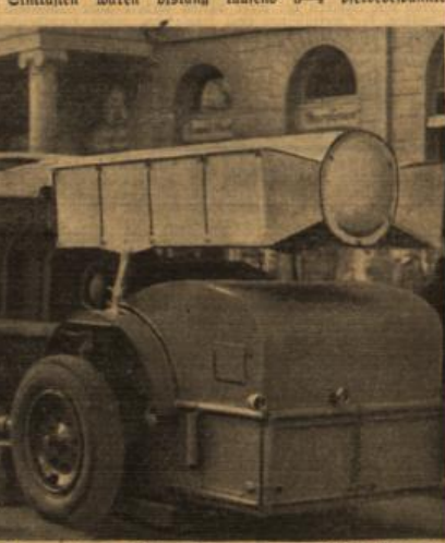
Die selbstausnehmende Kehrmaschine mit Staubfangvorrichtung. (Foto: Ebert.)
