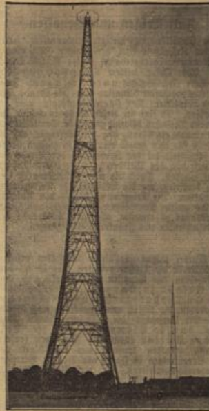
Der Sendeturm in Langenberg eingestürzt. (Deutsche Presse-Photo-Zentrale, M.)
