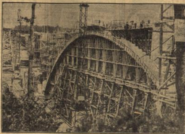
Die größte Eisenbetonbrücke Deutschlands geht ihrer Vollendung entgegen.
