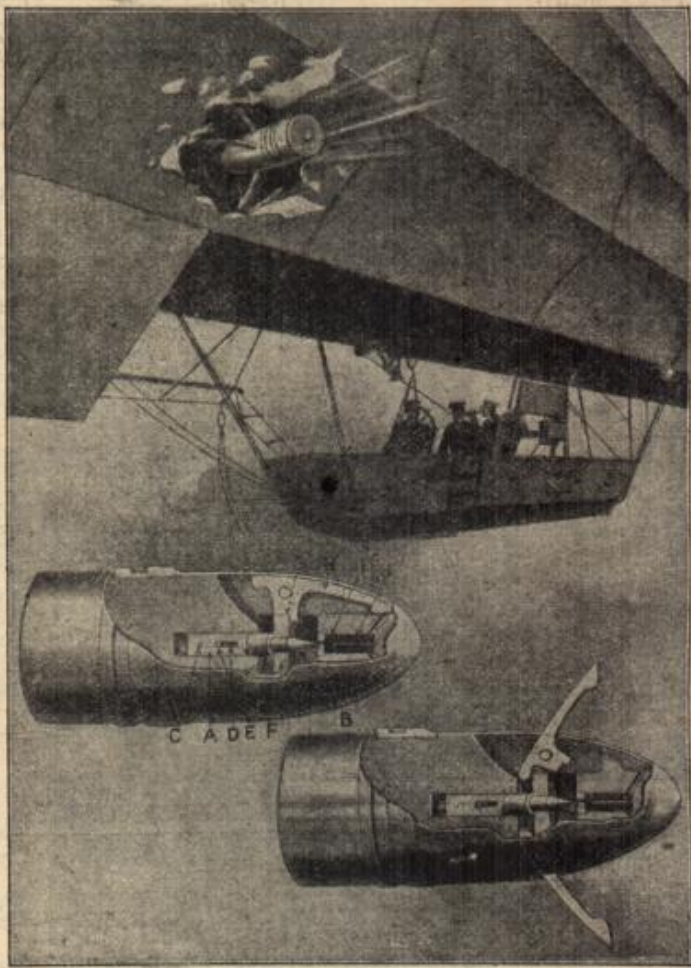
Explosivgeschloß zur Vernichtung von Luftschiffen. (Mit Text.)
