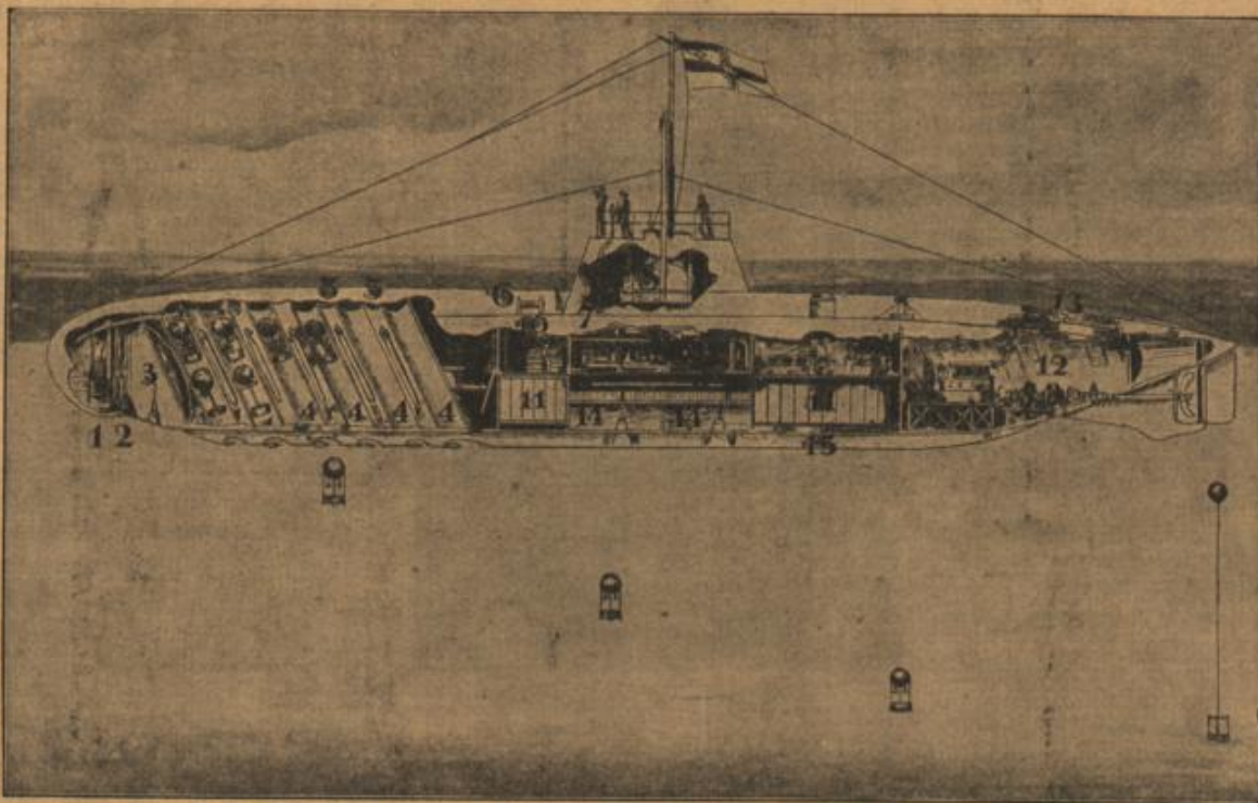
Deutscher Tauchboot-Minenerleger. (Ziffernerklärung siehe den Text.)
