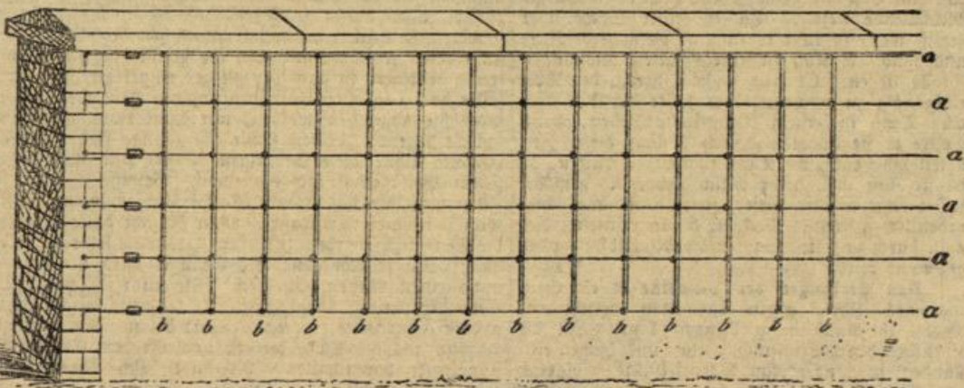
Abbildung 5. Anbringen eines Spaliergerüsts. a verzinkte Stenndrähte, Entfernung voneinander 50 bis 60 cm. b Spalierlatten ober Lattenfläche (Entfernung 50 cm).
