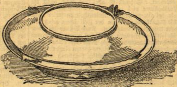
Abbildung 2. Teller-Keimprobe (bedeckt).
