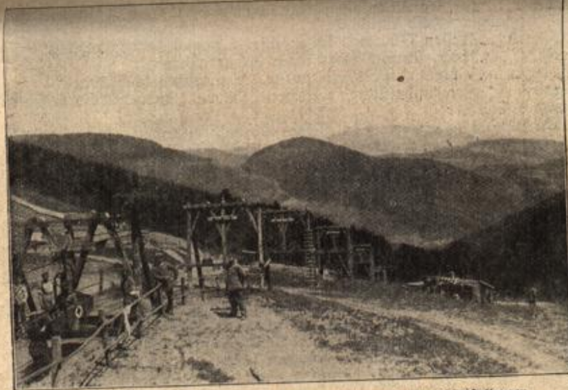
Trichtseilbahn zur Beförderung von Verwundeten aus den Höhenstellungen.
