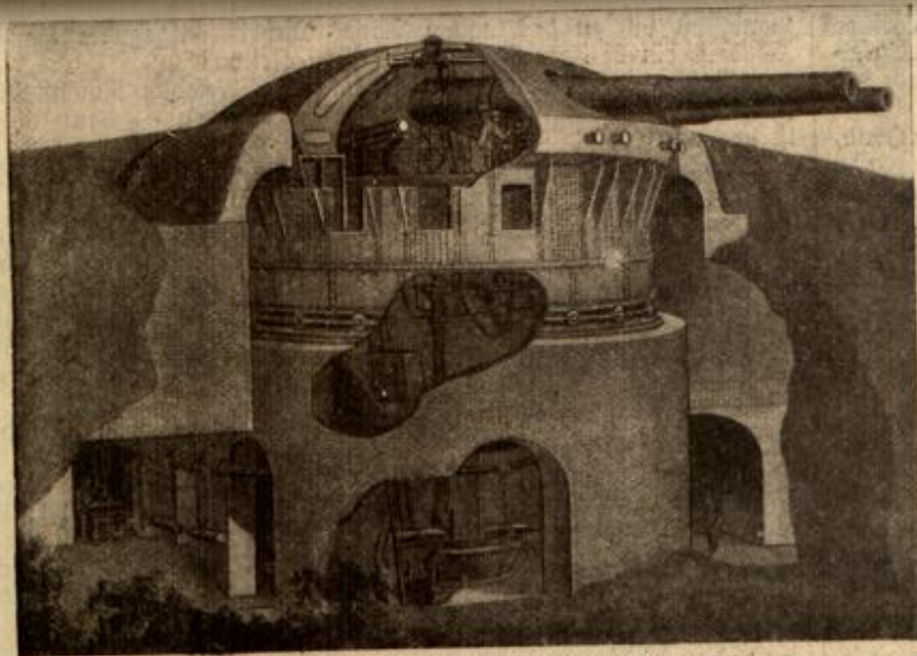
Durchschnitt durch einen französischen Panzerthurm.
