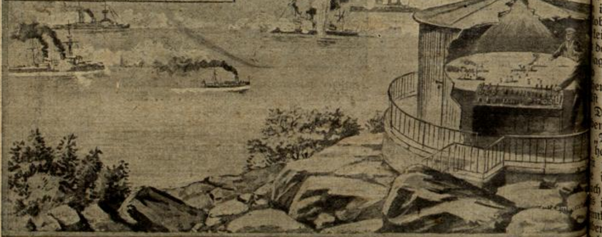
Darstellung einer Hafensperre durch Beobachtungsmineen. (Mit Text.)
