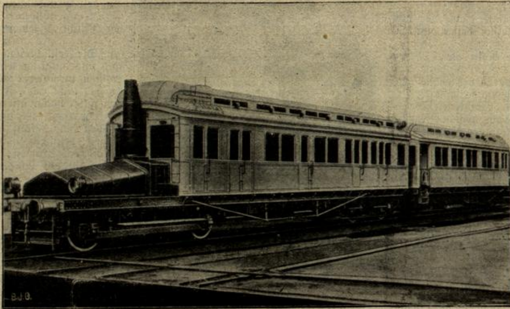
Der neue benzol-elektrische Hofzug des Khediven von Agypten. (Mit Text.)
