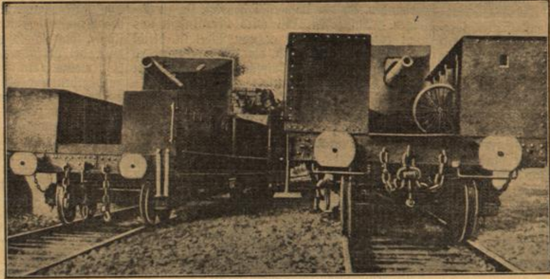
Schwere gepanzerte englische Geschützwagen, die im nordwestlichen Frankreich Verwendung finden. Der eine Wagen links hat den Namen „Big Willie“ und der andere „Little Willie“.
