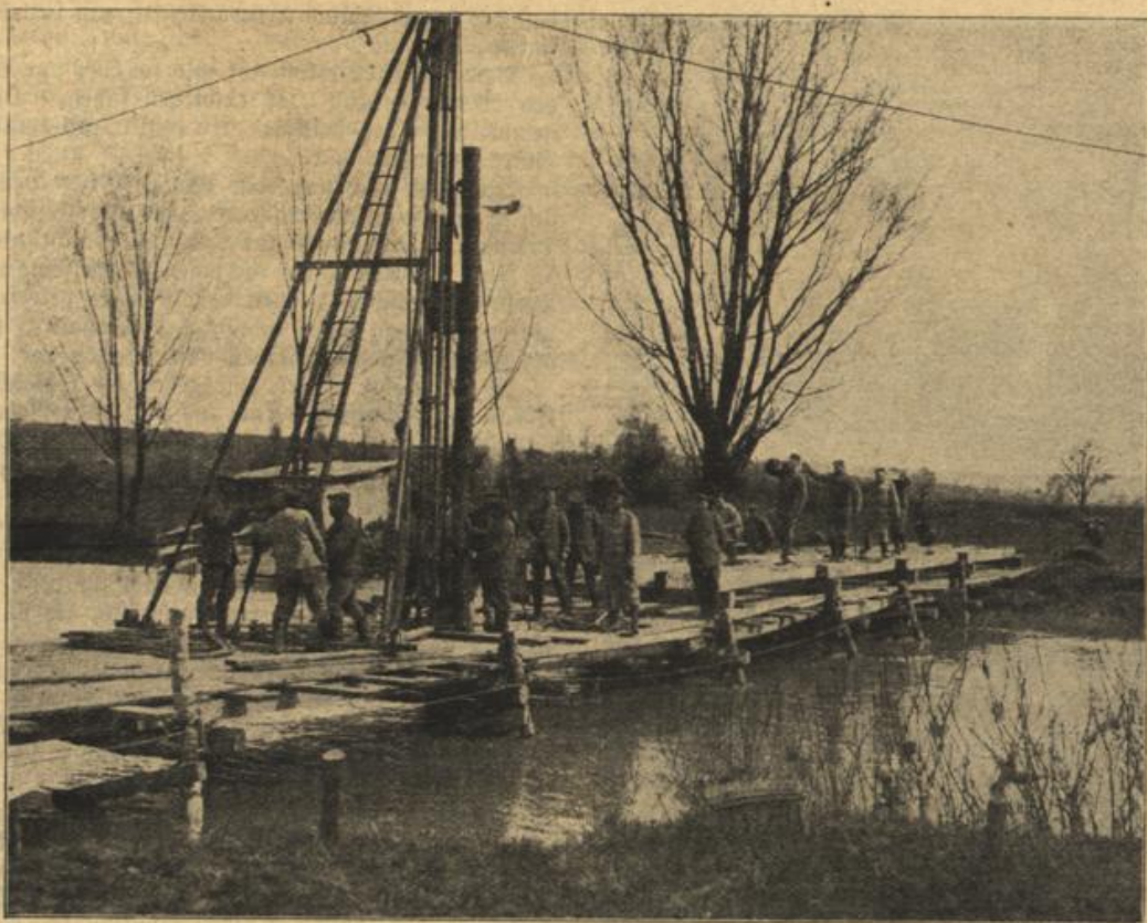
Pioniere beim Brückenbau.
