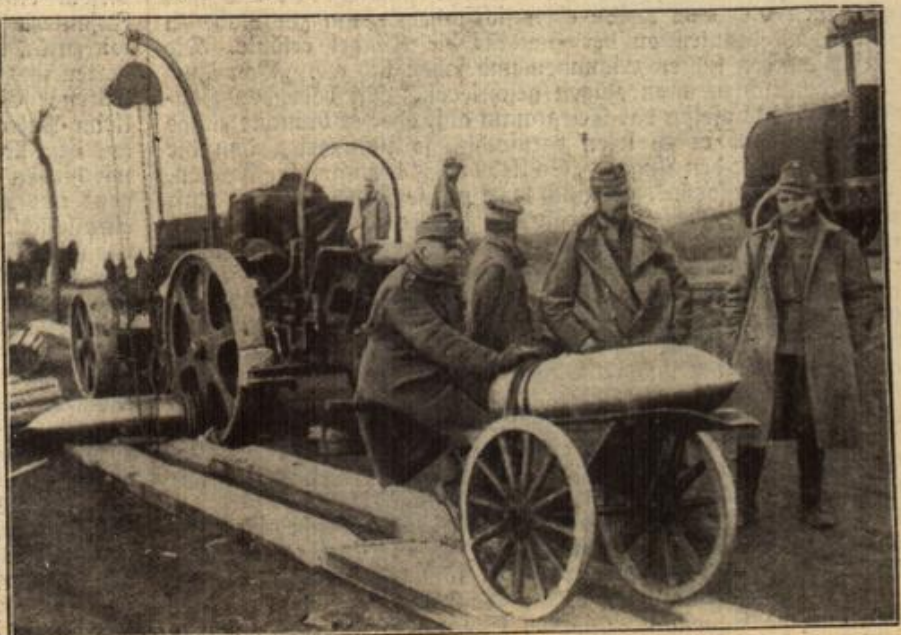
Geschosswagen der österr. 30,5 cm-Motormörser mit einem Geschos. (Mit Text.)
