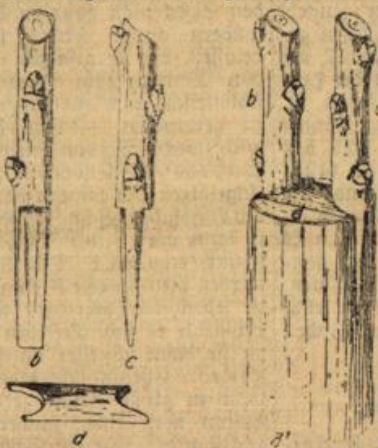
Abbildung 2. Das Pfropfen in den ganzen Spalt bei schwächeren Ästen. a) Edelreis (Borders- und Seitenansicht), b) Rinden-Decken der Spaltwunde, a') die Reiser aufgesetzt.
