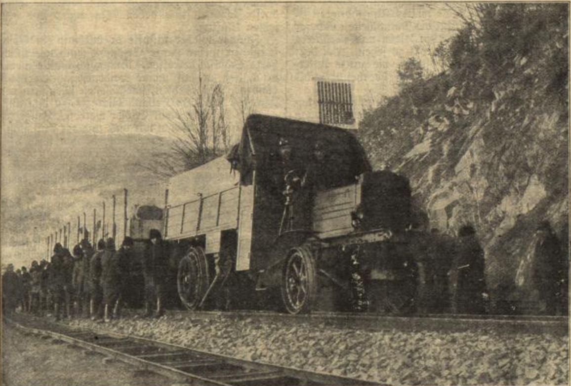
Osterreichisch-ungarisches Lastautomobil auf Schienen als improvisierte Feldbahn in den Karpathen. Phot. K. K. Hofphot., Wien.
