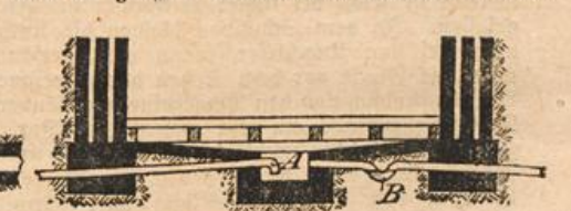
Abbildung 3. Ableitung des Eis-Schmelzwassers in undurchlässigem Untergrund.
