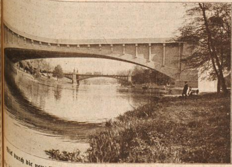
Die neue Eisenbahnbrücke auf die König-Karls-Brücke in Cannstatt. Emil Nicolai, Cannstatt, phot. (Mit Text.)
